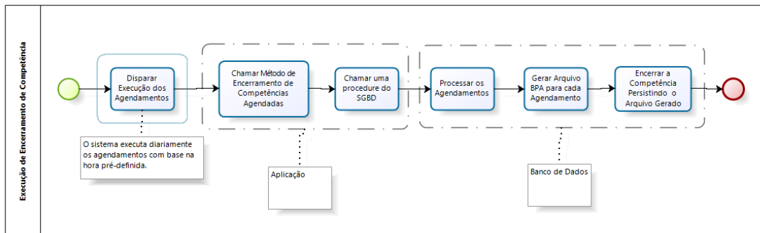
Figura 6 – Processo de Execução do Encerramento de Competência
